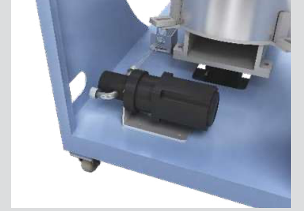
Yüksek Hassasiyetli Sıvı Dişli Pompası
